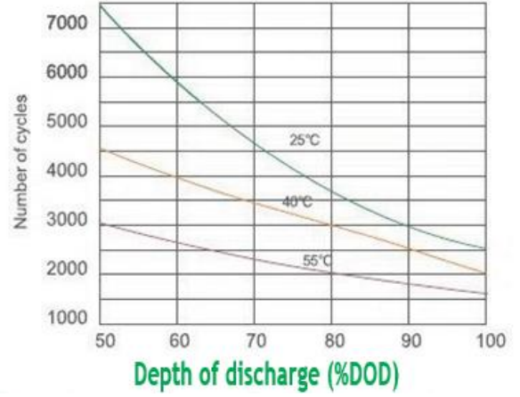
Farklı Sıcaklık Deşarj Eğrisi (0.2C)
