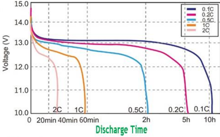
Farklı Hızda Deşarj Eğrisi
