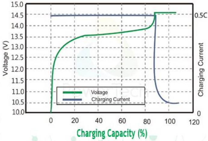
Şarj Karakteristikleri @ 0,5C 25°C
