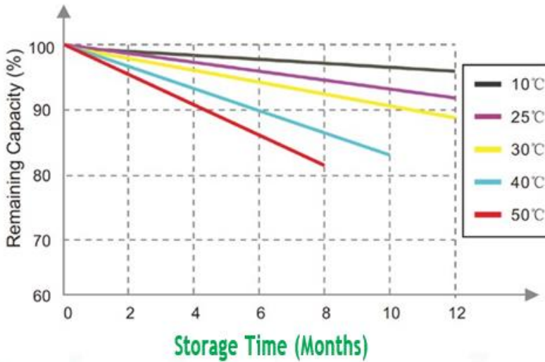
Şarj Durumu Eğrisi @0.5C 25°C
